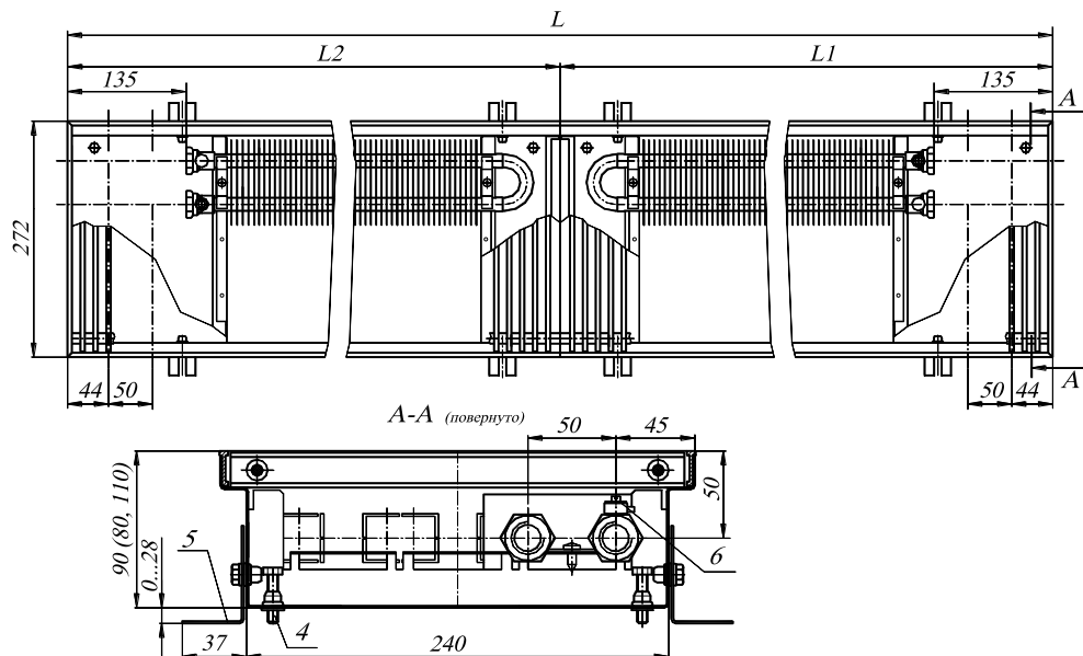
Рис. 3 Конвектор КРК 27.08(09,11) 320...600 – ЛП
