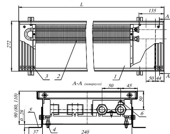
Рис. 1 Конвектор КРК 27.08(09,11).60...310 - П 1 - корпус установочный; 2 - элемент нагревательный; 3 - решетка; 4 - болты упорные; 5 - кронштейны; 6 - клапан воздушоспускной;
